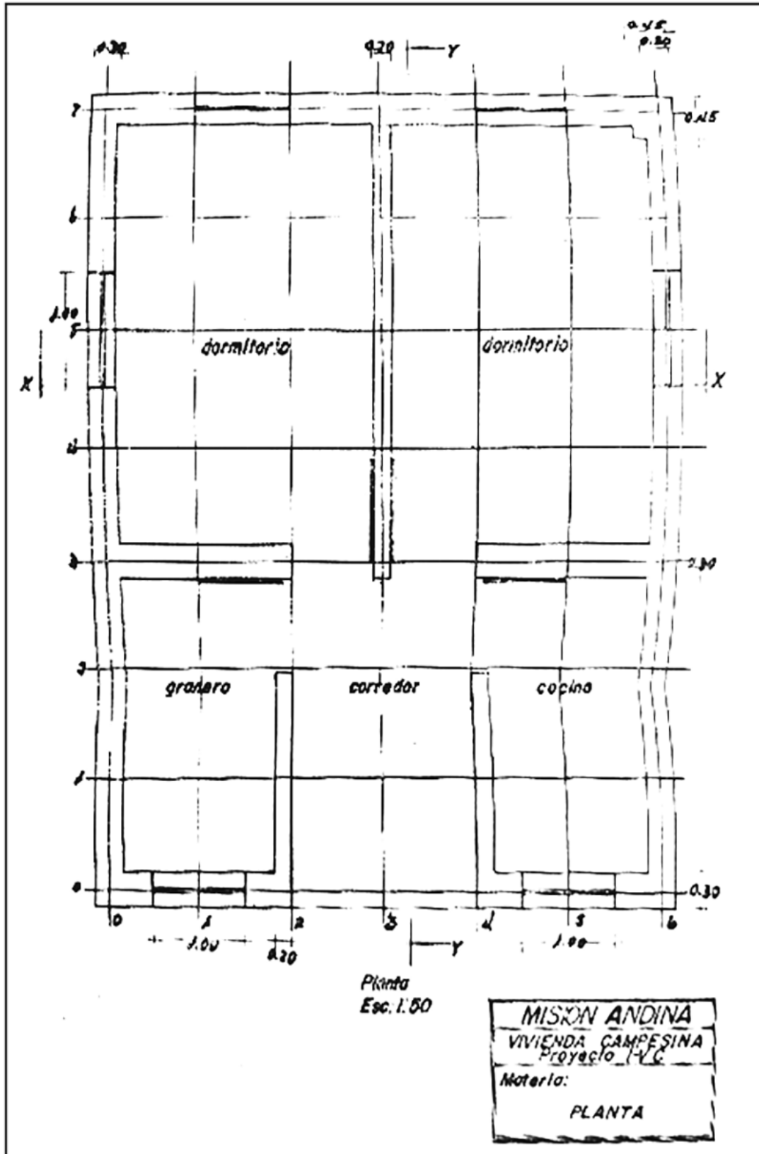
Figura 5. Plano del prototipo de vivienda mejorada.
